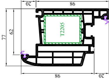
T2205 Ouvrant Z78 - 544725 Renfort : TS107 - TS131 - TS130
