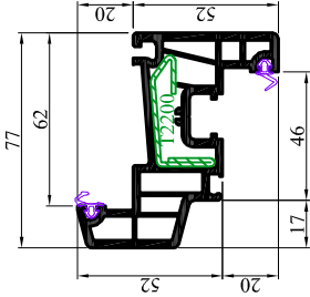
T2200 Ouvrant Z52 - 555848 Renfort : TS101 - TS111
