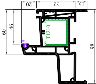
T1210 Dormant 98 - 540095 Renfort : T5004 - T5014
