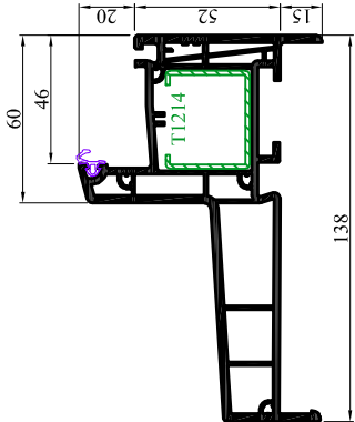
T1214 Dormant 138 - 540135 Renfort : T5004 - T5014
