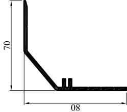
T1800 Habillage de 70*80 mm - 561401
