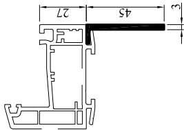
T1810 Habillage de 45 mm - 758370
