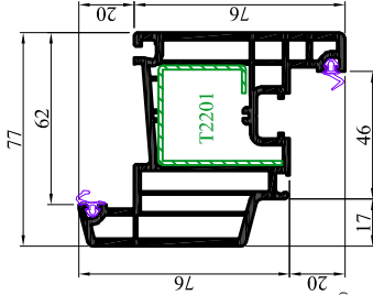
T2201 Ouvrant Z76 - 548865 Renfort : TS102 - TS112 - TS120
