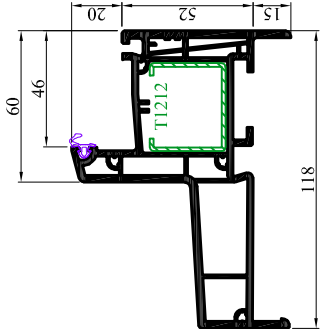
T1212 Dormant 118 - 540115 Renfort : T5004 - T5014
