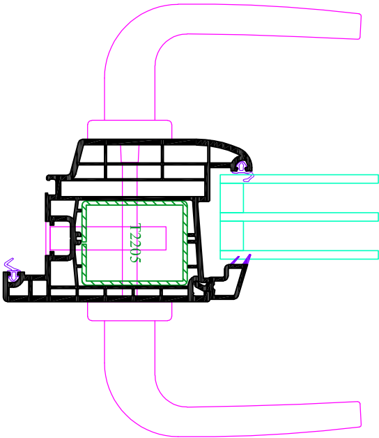
Fouillot de 40 mm
