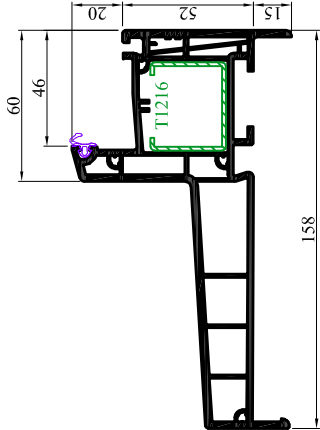
T1216 Dormant 158 - 540155 Renfort : T5004 - T5014
