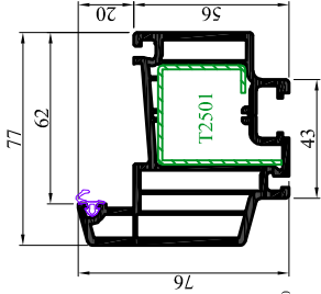
T2501 Battement B076 - 548875 Renfort : TS102 - TS112 - TS120
